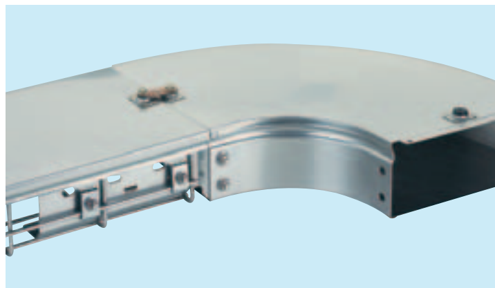
2 Сборка соединения F31 на металлическом лотке
