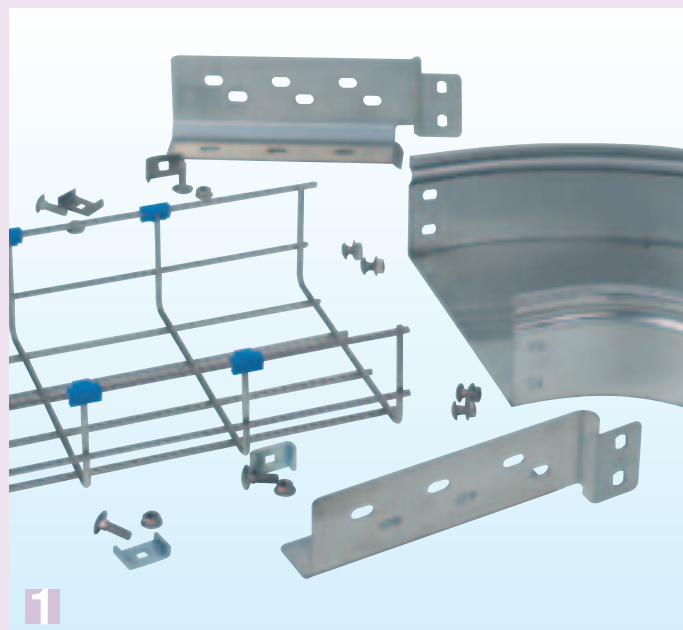
1 Соединение F31 в разобранном виде
