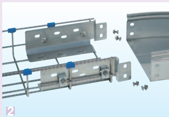
2 Сборка соединения F31 на металлическом лотке
