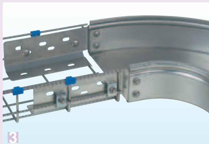
3 Выравнивание элементов и затяжка. Рекомендуется использовать две точки затяжки на каждое соединение на боковой стороне F31
